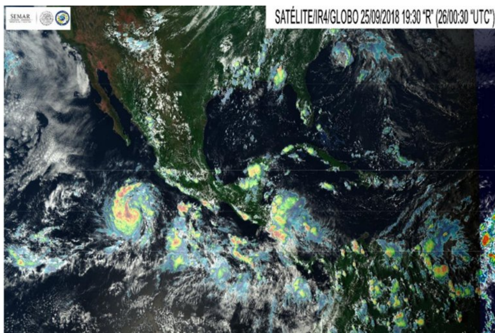
Figura 34. Imagen de satélite de las 19:30 horas “R” del 25 de septiembre, se puede ver a la Tormenta Tropical “Rosa” con sus bandas nubosas de gran cobertura espacial.
