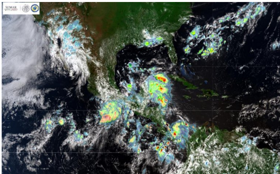
Figura 7. Imagen de satélite donde se observa la disipación de Bud sobre el Golfo de California, así como sus bandas nubosas (Imagen proporcionada por el CAPMAR).
