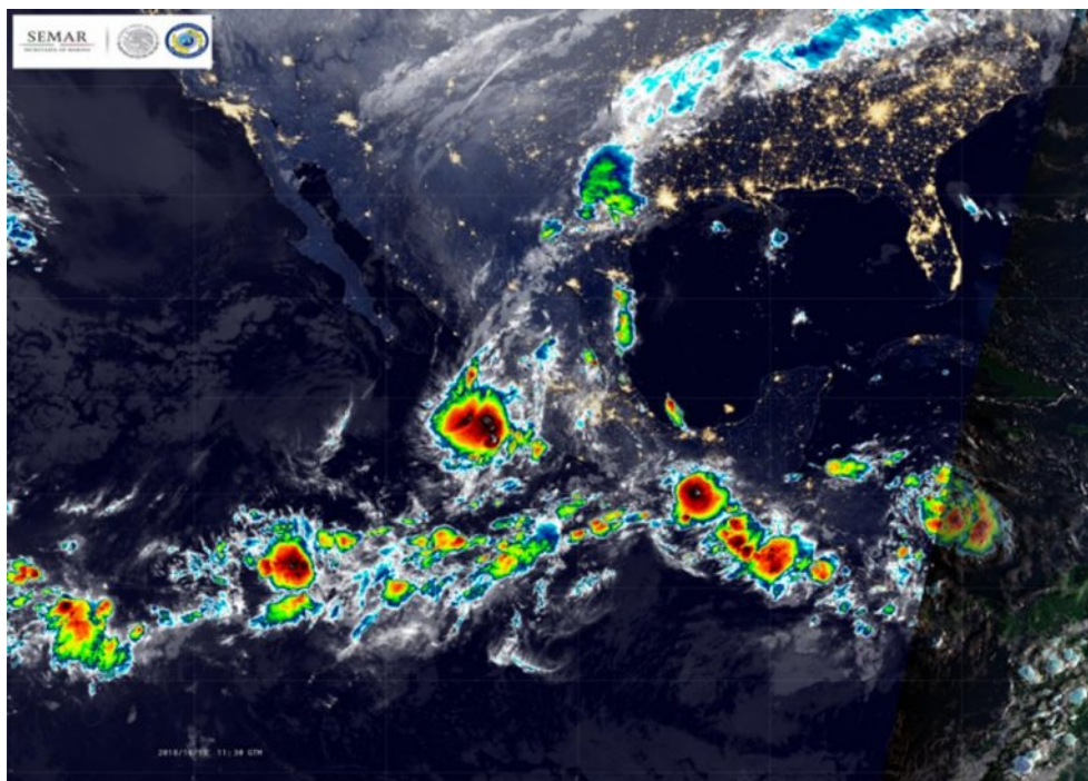
Figura 39. Imagen satelital de las 06:30 horas “R” del 15 de octubre, donde se observa a la Tormenta Tropical “Tara” (Proporcionado por el CAPMAR).
