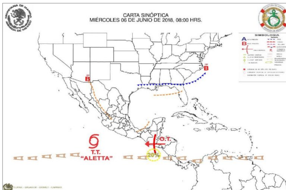
Figura 1. Ubicación de la Tormenta Tropical “Aletta” en el Pacífico central mexicano el día 06 de junio. (Carta sinóptica elaborada por el CAPMAR).
