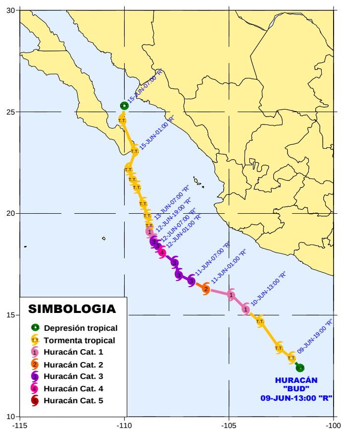
Figura 8. Trayectoria del Huracán "Bud" Categoría-4, del 09 al 15 de junio (Elaborado por el Departamento de Climatología con datos de Unisys Weather).
