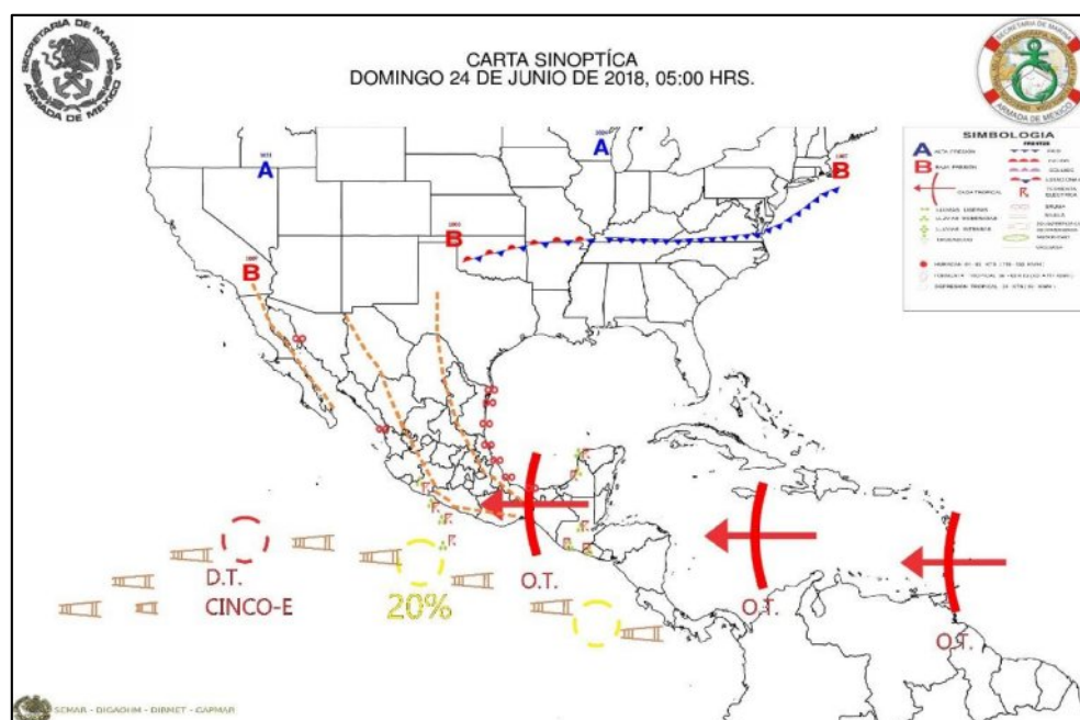
Figura 12. Mapa sinóptico donde se observa la Depresión Tropical “Cinco-E” , fuera de la Zona Económica Exclusiva el 24 de junio a las 05:00 horas “R” (Elaborada y proporcionada por el CAPMAR).
