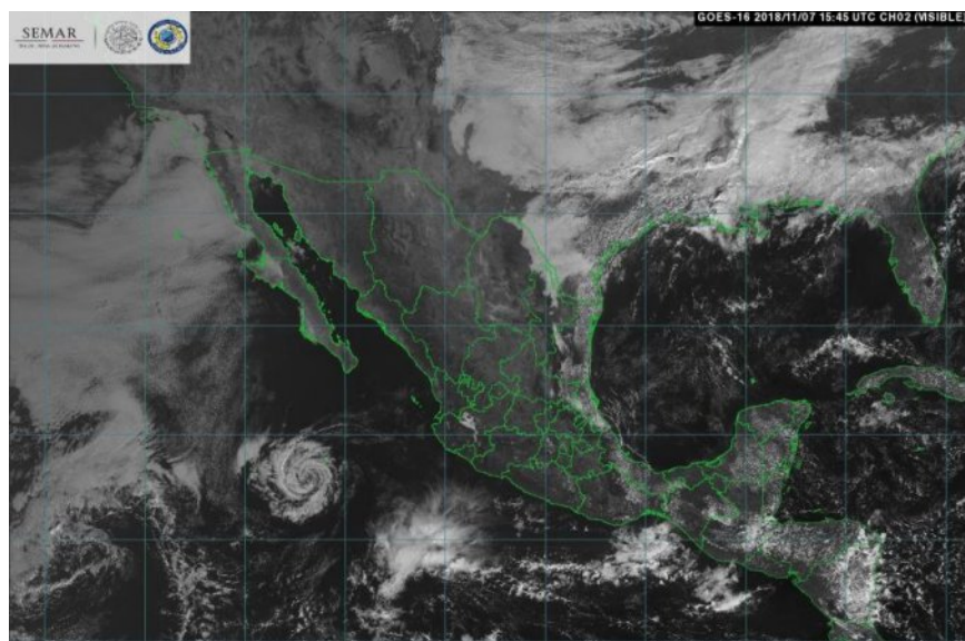
Figura 47. Imagen satelital en canal visible que corresponde al 07 de noviembre a las 09:45 horas "S", se observa a la Tormenta Tropical "Xavier" , dos días después de que la emitieran como disipada.
