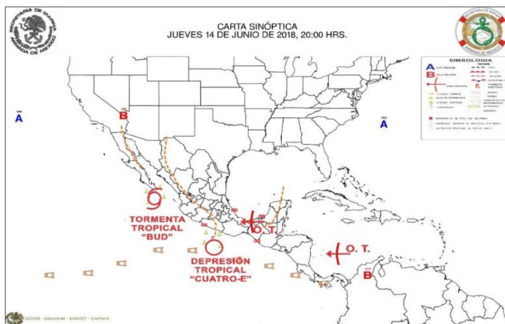
Figura 9. Carta sinóptica donde se observa a la Depresión Tropical “Cuatro-E” frente a la costa de Guerrero y los fenómenos meteorológicos que provocó (Elaborada y proporcionada por el CAPMAR).
