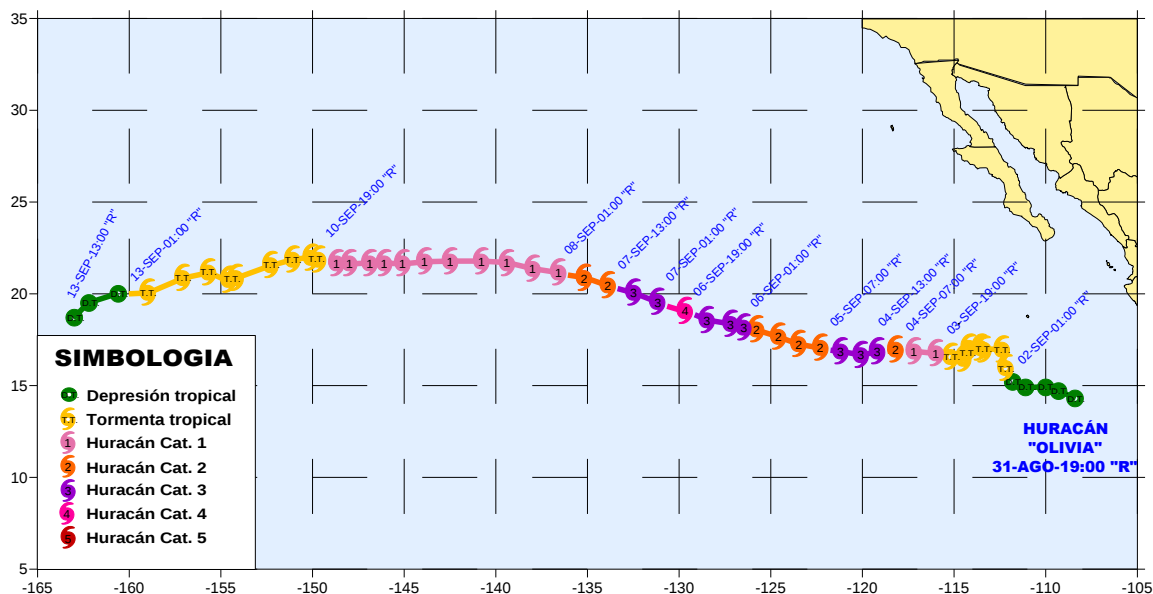
Figura 30. Trayectoria del Huracán "Olivia" Categoría-4 del 01 al 13 de septiembre (Elaborado por el Departamento de Climatología con datos de Unisys Weather).
